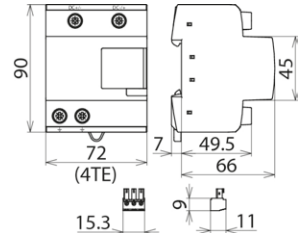
Maßbild DCB YPV 1500 FM
