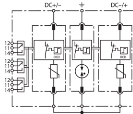
Principalschaltbild DG ME DC Y 950 FM
