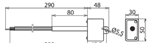
Maßbild DCOR L 2P 275 SO IP
