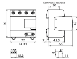
Maßbild DV M2 TT 255 FM
