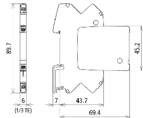
Maßbild BCO ML2 B 180
