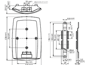
Maßbild DPA CLE IP66
