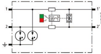
Prinzipschaltbild BCO ML2 BD HF 24
