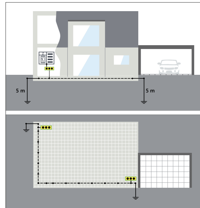
Erdungsanlage mit Tiefenerder für Wohngebäude ohne Keller
