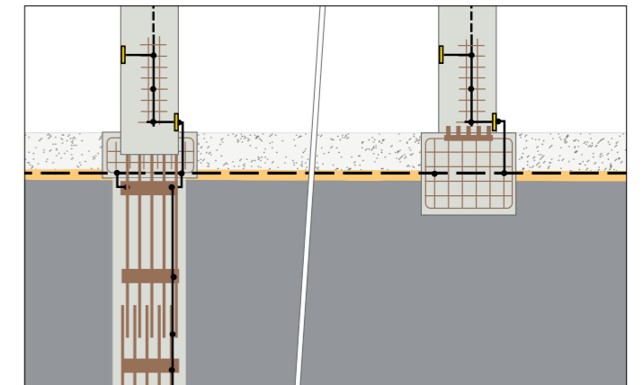
Bautechnische Ausführung von Einzelfundamenten
