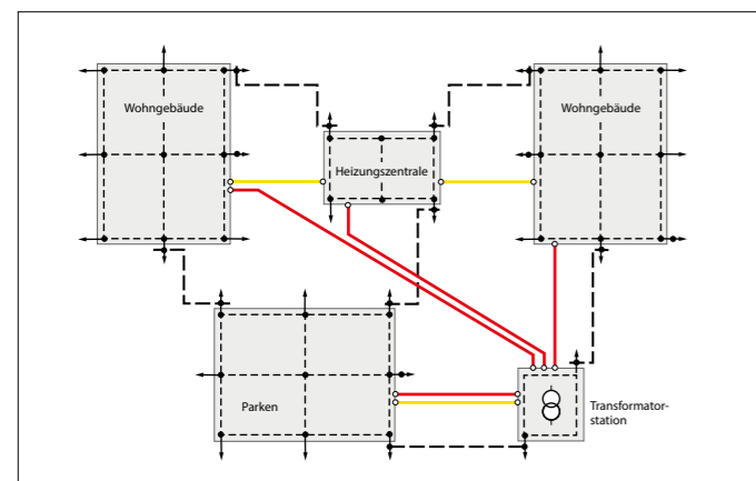
Vermaschte Erdungsanlage bei Industrieanlagen
