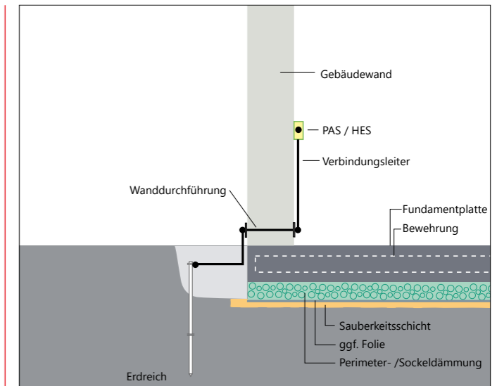
Praktische Ausführung Tiefererder ohne Keller
