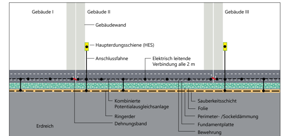
Praktische Ausführung Ringerder und CBN
