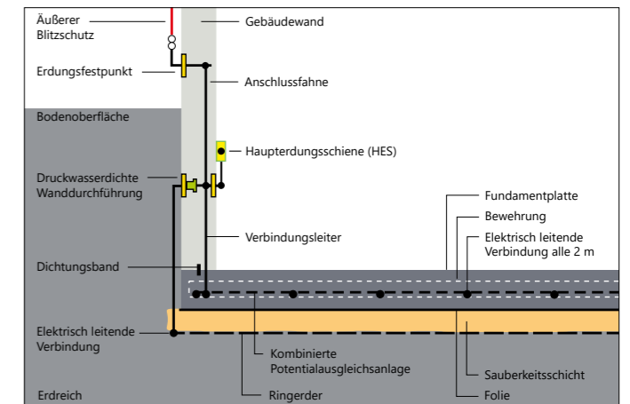
Praktische Ausführung Ringerder und CBN
