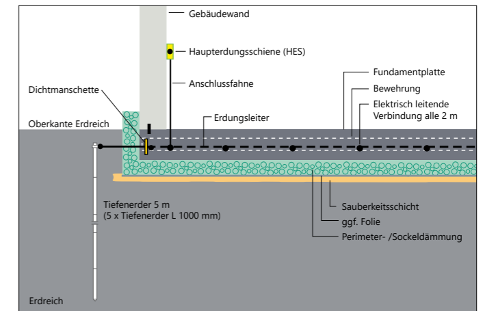
Praktische Ausführung mit Tiefenerder
